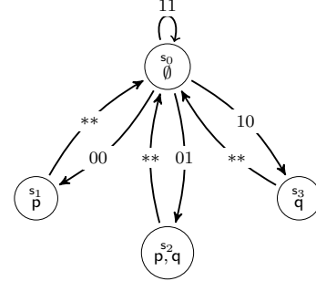
Fig. 4: The CGS \mathcal{G}_{SV} .
