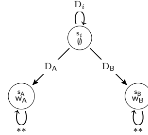
Fig. 1: The CGS \mathcal{G}_{PRS} .
