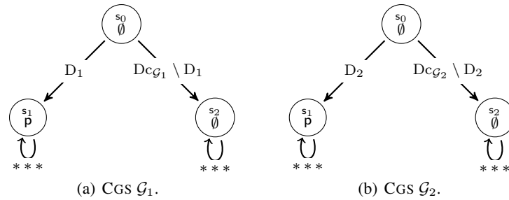
Fig. 7: Alternation-2 non-equivalent CGSs.
