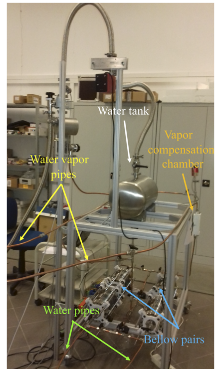
FIG. 4. LAG liquid handling system.
