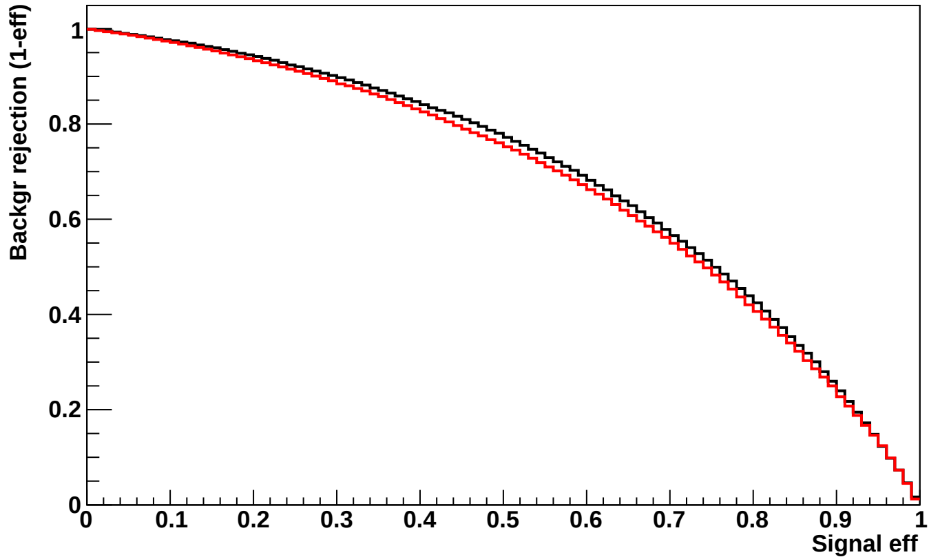
MVA_LikelihoodMIX
