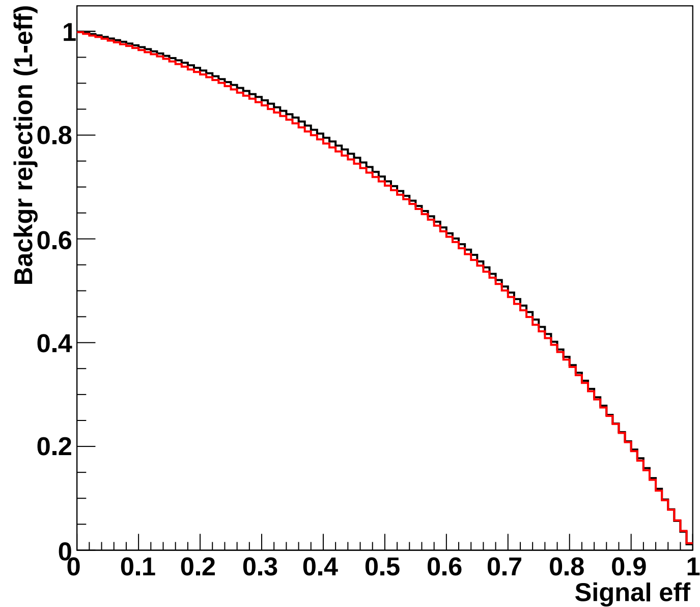
MVA_LikelihoodMIX
