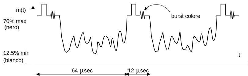
Forma d'onda del segnale televisivo
