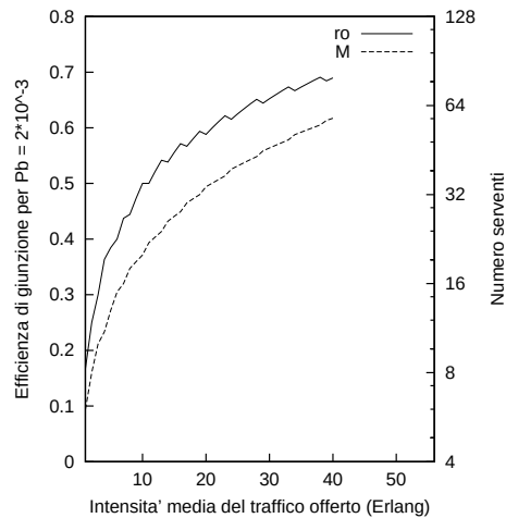
Figura 6.2: Andamento dell'efficienza \rho e del numero di serveri per una probabilità di blocco P_B prefissata
