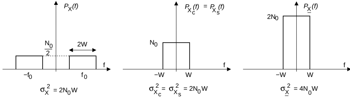
Figura 8.2: Densità di potenza per rumore passabanda
