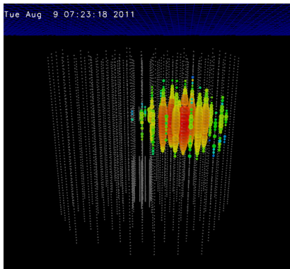
“Bert” \sim 1050 TeV
