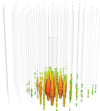
82.2 TeV, -13^\circ
