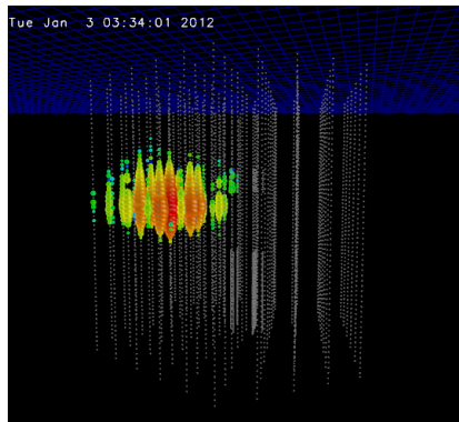
“Ernie” \sim 1150 TeV arXiv:1304.5356
