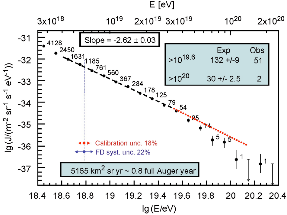
Figura 1.12: Misure dello spettro dei raggi cosmici alle energie più alte ottenuto dalle osservazioni di Auger [Auger Collaboration (2008)].
