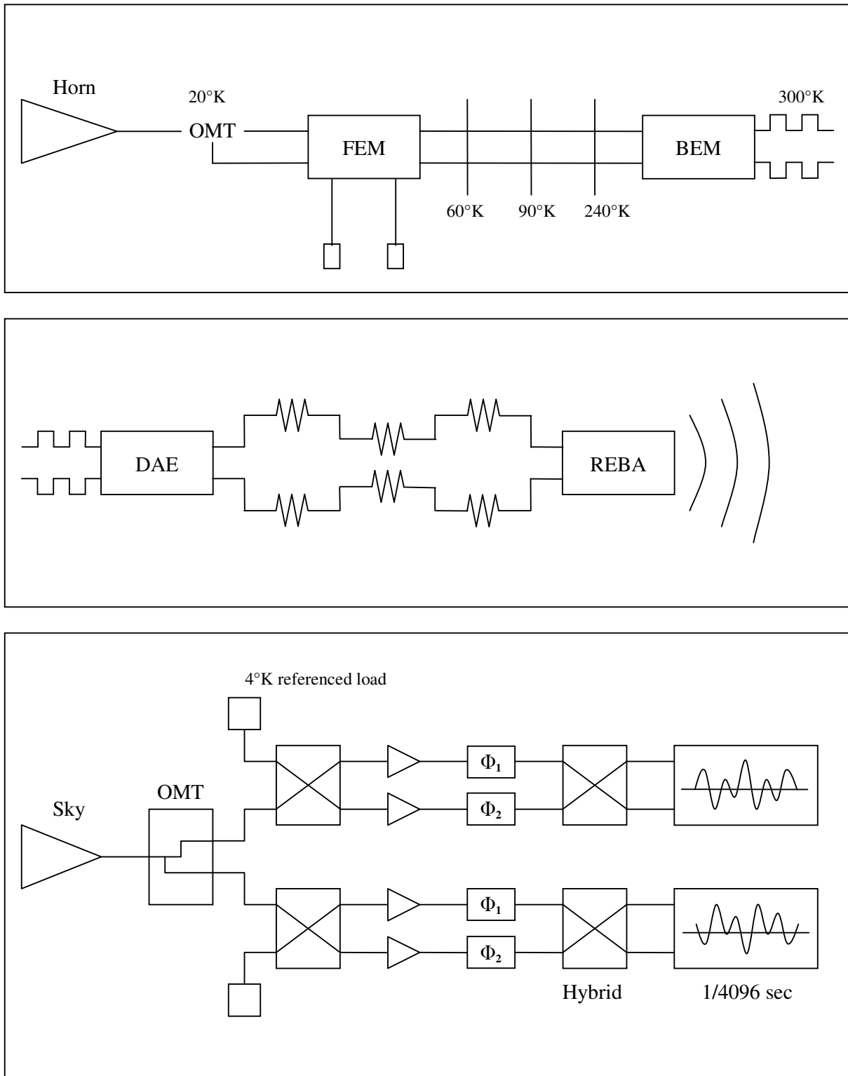
Figura 34: Schemi circuitali di LFI
