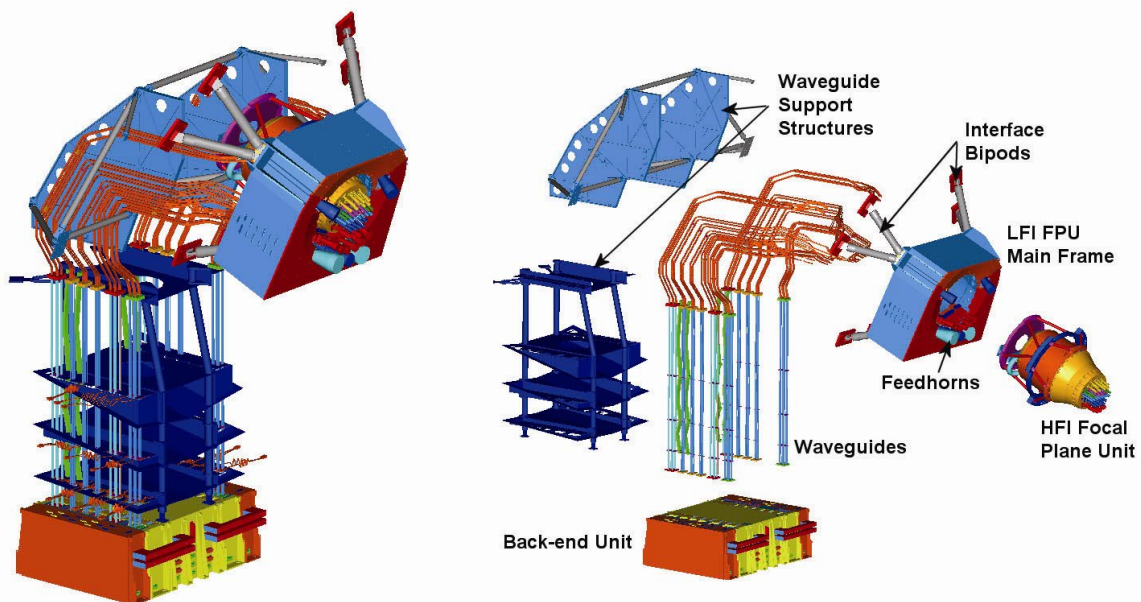
Figura 30: Struttura degli strumenti di Planck
