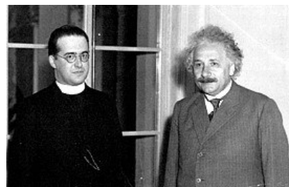
Figura 2: Lemaître e Einstein
