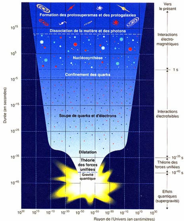
Figura 26: Nascita dell'Universo
