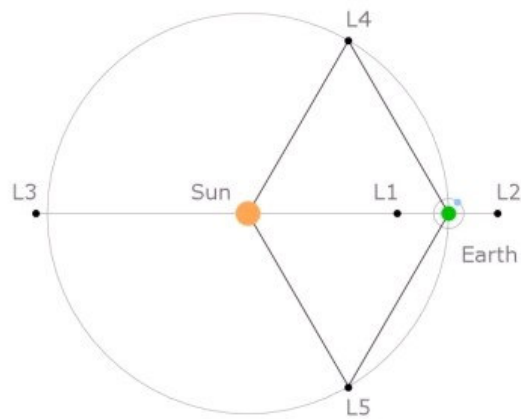
Figura 10: Orbita L2
