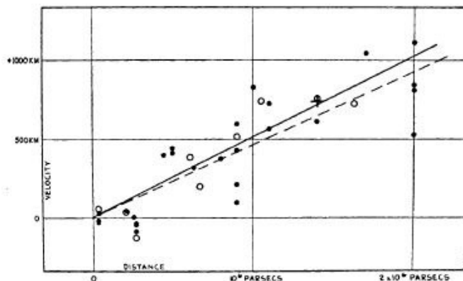
Figura 20: Legge di Hubble
