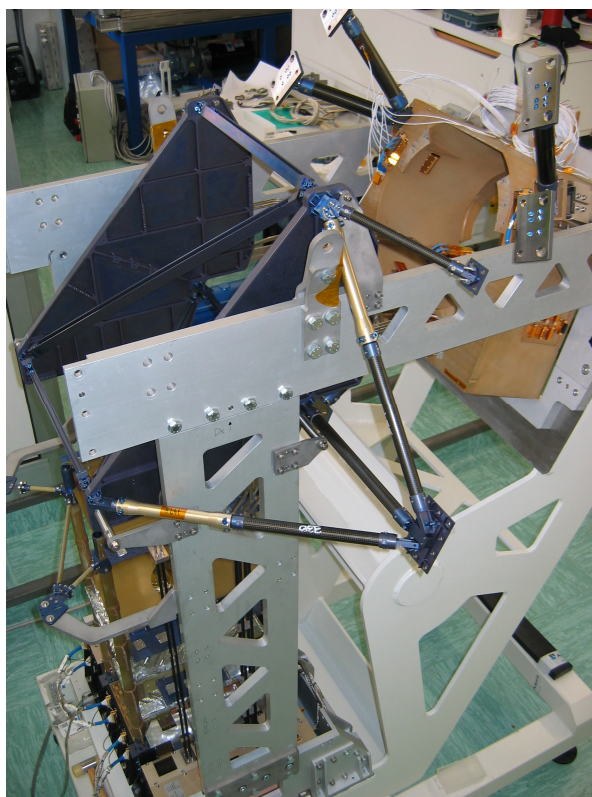
Figura 41: Struttura LFI
