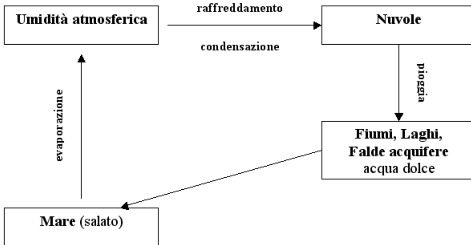
Ciclo dell'acqua
