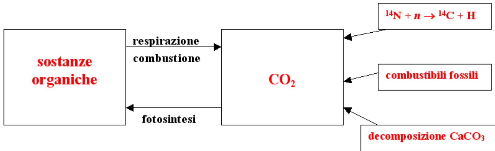
Ciclo del carbonio
