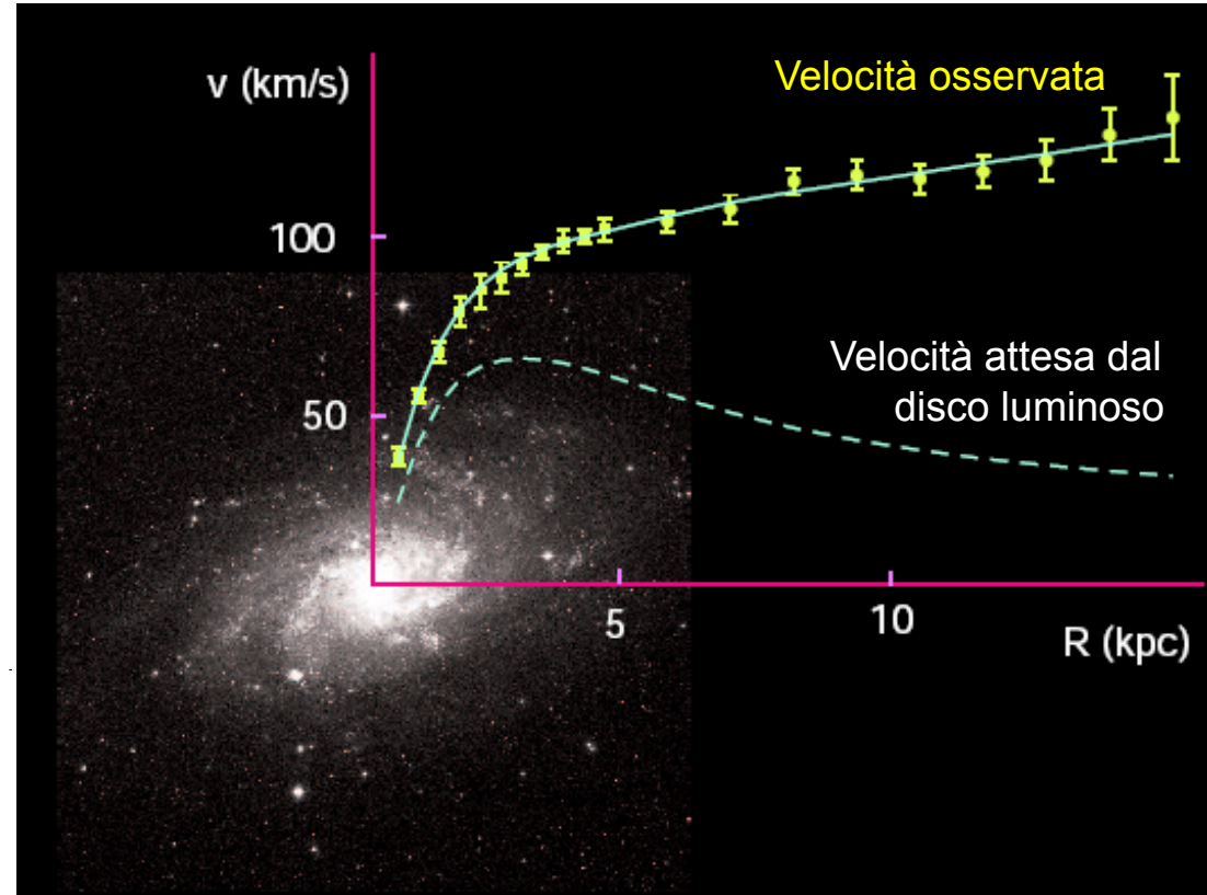
Curva di rotazione della galassia M33
